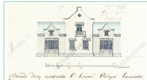
И. И. Антонов (по образцовому проекту А. И. Штакеншнейдера). Фасад дома чиновника 6-го класса Камкова (по Головкинской, ныне Конюшенной, улице). 1837 г.
